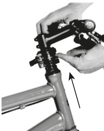
Figura 40: Sollevamento della leva di sicurezza, esempio by.schulz speedlifter
