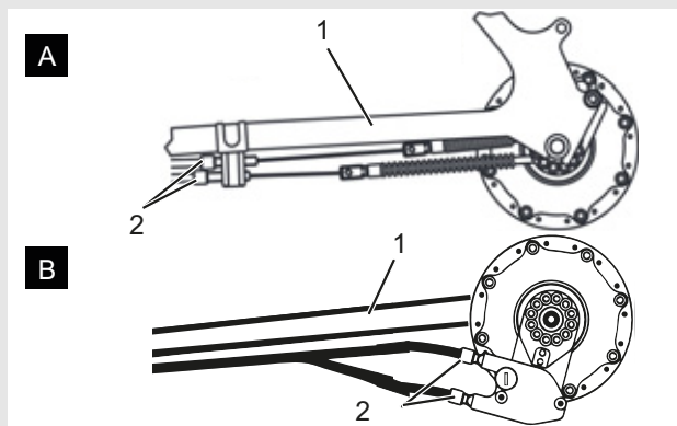
Figura 69: Boccole di regolazione (2) di due versioni alternative (A e B) di un cambio azionato da cavo doppio sul fodero orizzontale (1)
