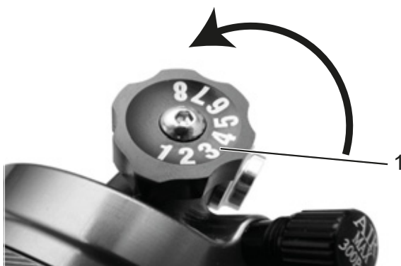
Figura 50: Regulador de niveles de presión Suntour en el amortiguador de la horquilla trasera
