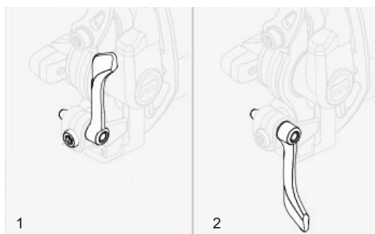
Figura 9: Palanca de bloqueo del freno de llanta, cerrada (1) y abierta (2)
