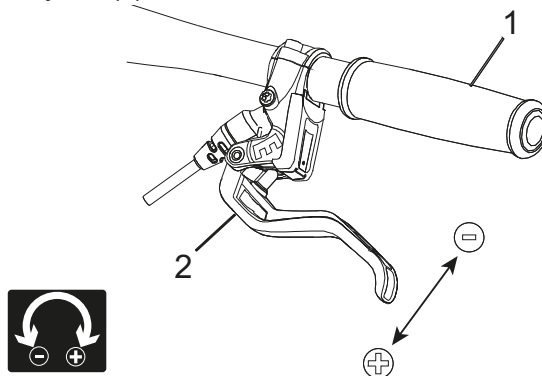
Figura 41: Ajustar el ancho de agarre de la palanca de freno Magura HS33
