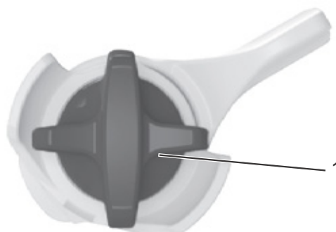
Figura 52: Regulador de niveles de tracción FOX (1) en el amortiguador de la horquilla trasera
